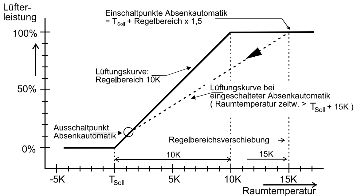
Bild 4: Absenkautomatik
