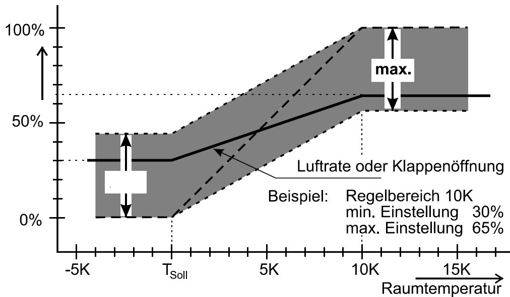
Bild 2: Einstellen der min. und max. Lüfterleistung bzw. Klappenöffnung
