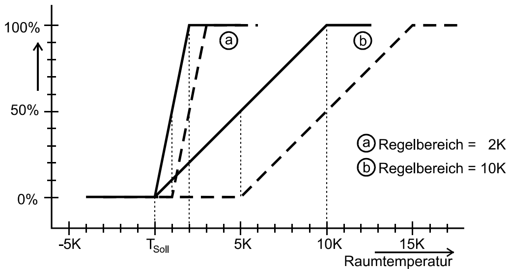
Bild 9: Regelversatz Im vorstehenden Diagramm ist die Auswirkung auf die Steuersignale bei einem Versatz von 50% des Regelbereichs dargestellt.
